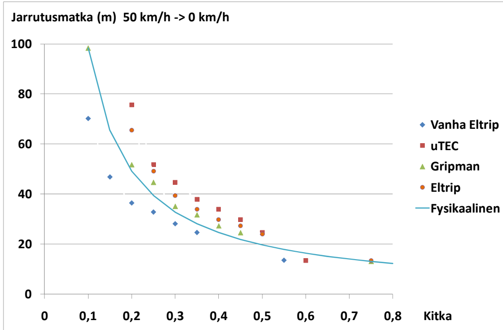
Kuva 20. Mitatun kitkan ja jarrutusmatkan yhteys testiratasteesteissä. Testeissä käytetyt jarrutusmatkat 40 km/h -> 5 km/h ja 50 km/h -> 5 km/h on muutettu laskennallisesti muotoon 50 km/h -> 0 km/h. Fysikaalinen kitka tarkoittaa fysiikan lakien mukaista jarrutusmatkaa eri kitkatasoilla. Jarrutusmatkat nopeudesta 80 km/h nopeuteen 0 km/h saadaan, jos kerrotaan pystyakselin luvut 2,5:llä.
