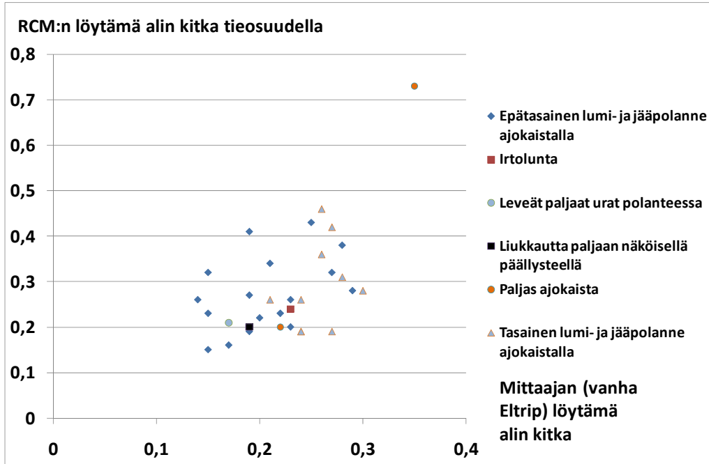
Kuva 39. RCM:n ja vanhan Eltripin vertailua pistokoelaadunseurannan yhteydessä sellaisilla tiejaksoilla, joilla vallitsi sama tienumero ja yhtenäinen keililuokitus. Mittauspäivät 7.3, 8.3. ja 13.3.
