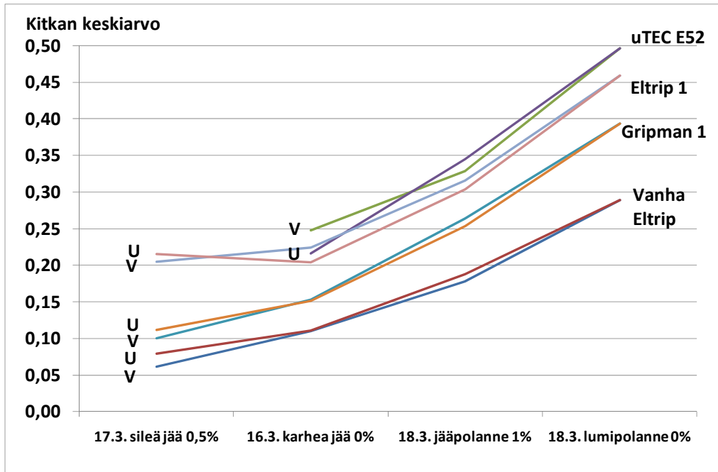
Kuva 24. Uusilla (U) ja vanhoilla (V) renkailla saavutetut kitkan keskiarvot, kun uusien renkaiden kitka-arvot on tätä analyysiä varten kalibroitu jälkeenpäin siten, että uusien renkaiden kitka vastaa vanhojen renkaiden kitkaa 18.3. lumipolanteella.
