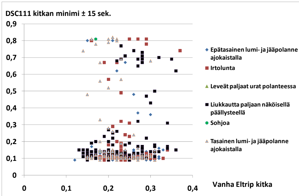
Kuva 42. DSC111:n ja vanhan Eltripin vertailua pistokoelaadunseurannan yhteydessä tehdyissä mittauksissa 24.3., 25.3., 28.3. ja 29.3. DSC111:n kitka on kitkan minimi ajanjaksona, joka on \pm 15 sekuntia vanhan Eltripin kitkanmittauksen ajanhetkestä.
