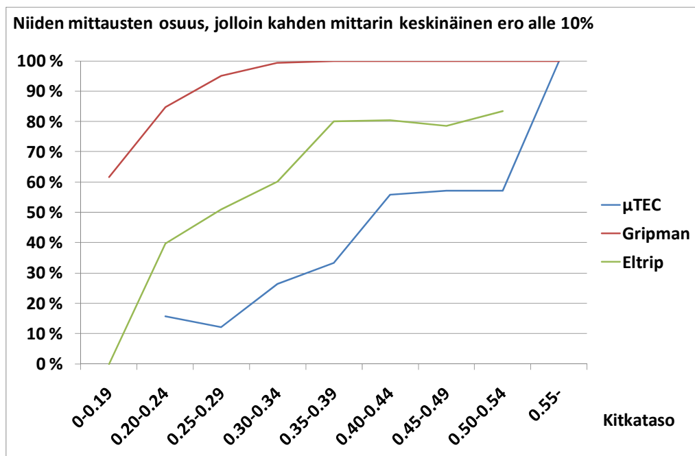
Kuva 46. Niiden mittausten osuus, jolloin saman valmistajan kahden mittarin keskinäinen ero oli alle 10 % pistokoelaadunseurannan yhteydessä tehdyissä mittauksissa. Kitkataso on alempaa kitkaa näyttäneen mittarin kitkataso ja keskinäinen ero on laskettu: (suurempi arvo - pienempi arvo) / pienempi arvo.
