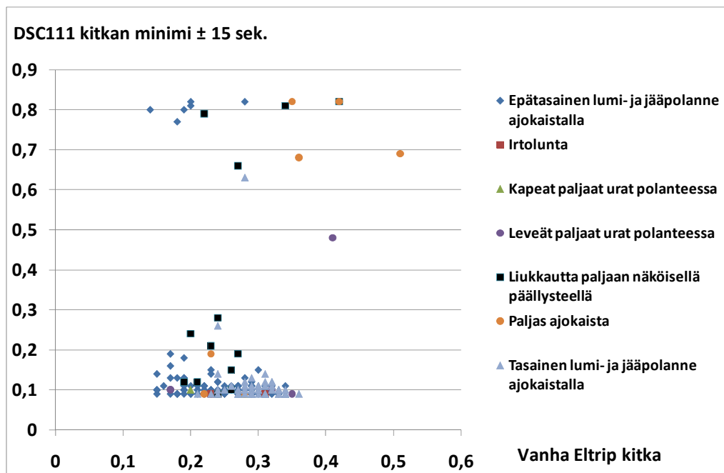
Kuva 41. DSC111:n ja vanhan Eltripin vertailua pistokoelaadunseurannan yhteydessä tehdyissä mittauksissa 7.3., 8.3. ja 13.3.. DSC111:n kitka on kitkan minimi ajanjaksona, joka on \pm 15 sekuntia vanhan Eltripin kitkanmittauksen ajanhetkestä.
