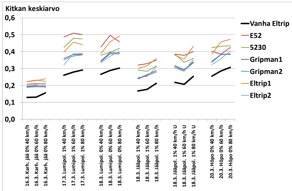
Kuva 21. Uusien kiihtyvyyssanturimittareiden ja vanhan Eltripin kitkan keskiarvo eri mittausnopeuksilla eri testiradoilla. radan kaltevuuden vaikutusta ei ole kompensoitu. Mittaukset on tehty sileällä jäällä sekä pinnoilla Pepo (pehmeä polanne), Kopo (kova polanne) ja Höpo (höylätty polanne) kumpaankin suuntaan. Muilla pinnoilla yhteen suuntaan. Jääpolanteella 18.3. mittauksia tehtiin myös uusilla renkailla (U), muuten mittaukset on tehty vanhoilla renkailla.
