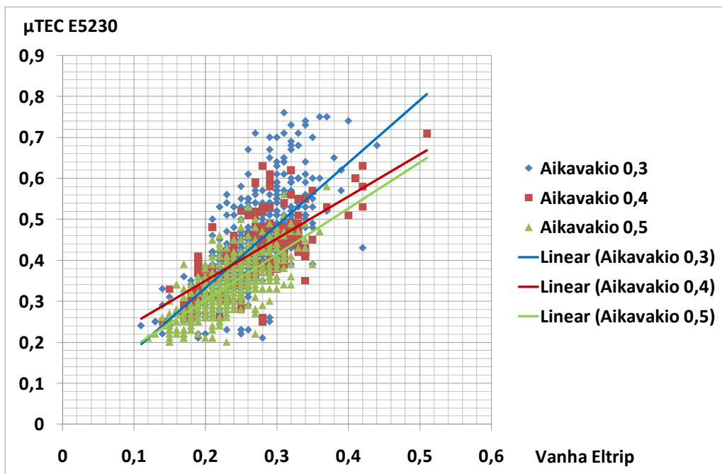
Kuva 32. 5230-matkapuhelimeen ladatun \mu TEC:in ja vanhan Eltripin vertailua. "Aikavakio 0,3" tarkoittaa ajanjaksoa 2.2.–28.2., jolloin \mu TEC:ien aikavakio oli 0,3. "Aikavakio 0,4" tarkoittaa ajanjaksoa 7.3.–13.3., jolloin aikavakio oli 0,4. "Aikavakio 0,5" tarkoittaa ajanjaksoa 24.3.–29.3., jolloin aikavakio oli 0,5. Tällä ajanjaksolla 5230-puhelin oli asetettu myös viinon E52 puhelimeen nähden.
