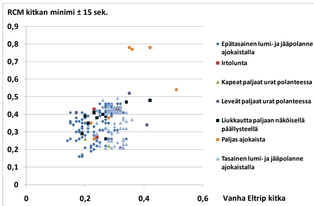
Kuva 38. RCM411:n ja vanhan Eltripin vertailua pistokoelaadunseurannan yhteydessä tehdyissä mittauksissa 7.3., 8.3. ja 13.3.. RCM411:n kitka on kitkan minimi ajanjaksona, joka on \pm 15 sekuntia vanhan Eltripin kitkanmittauksen ajanhetkestä.
