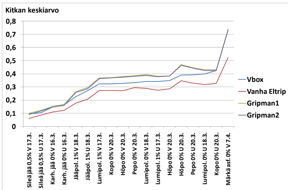
Kuva 17. Gripmanien ja Vanhan Eltripin sekä jarrutusmatkamittauksen (Vbox) perusteella laskettujen kitkojen keskiarvot eri testiradoilla. Jarrutusmatkamittauksissa on kompensoitu kaltevuuden vaikutus, mutta muilla laitteilla ei. Mittaukset on tehty sileällä jäällä sekä pinnoilla Pepo (pehmeä polanne), Kopo (kova polanne) ja Höpo (höylätty polanne) kumpaankin suuntaan. Muilla pinnoilla yhteen suuntaan. U=uudet renkaat, V=vanhat renkaat.
