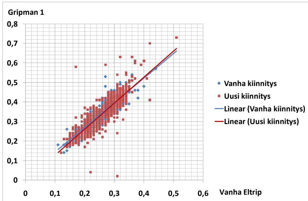
Kuva 33. Gripman 1:n ja vanhan Eltripin vertailua. "Vanha kiinnitys" tarkoittaa 2.2. ja 3.2. testeissä käytettyä kiinnitys, jossa Gripmanit oli sijoitettu hieman epävakampiin telineisiin. "Uusi kiinnitys" tarkoittaa 8.2.–29.3. käytettyä kiinnitystä, jolloin Gripmanit oli sijoitettu jäykempiin telineisiin.
