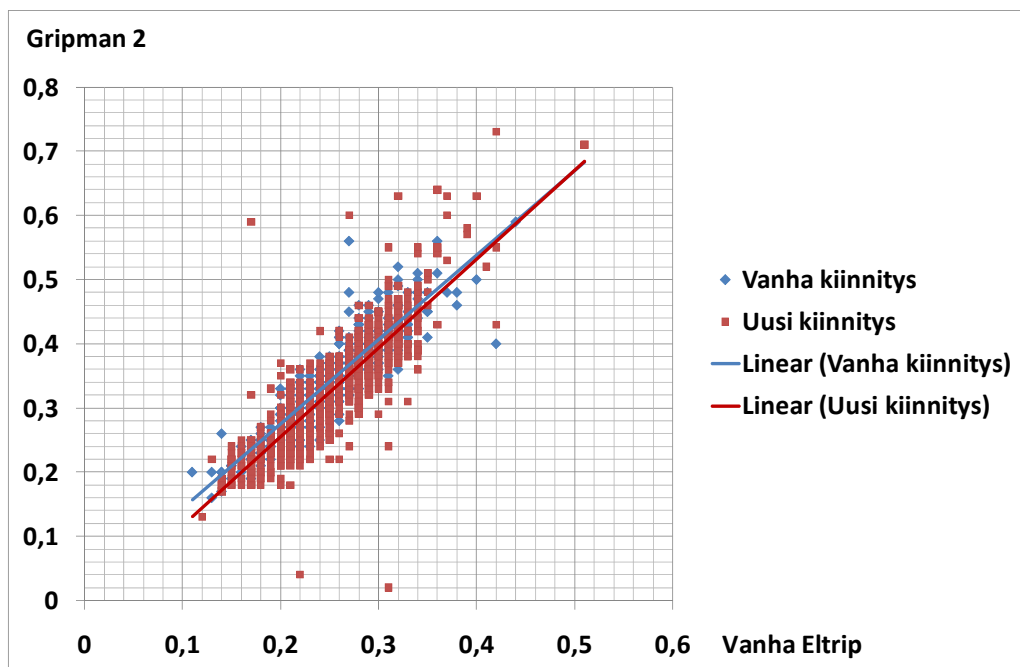
Kuva 34. Gripman 2:n ja vanhan Eltripin vertailua. "Vanha kiinnitys" tarkoittaa 2.2. ja 3.2. testeissä käytettyä kiinnitystä, jossa Gripmanit oli sijoitettu hieman epävakampiin telineisiin. "Uusi kiinnitys" tarkoittaa 8.2.–29.3. käytettyä kiinnitystä, jolloin Gripmanit oli sijoitettu jäykempiin telineisiin.
