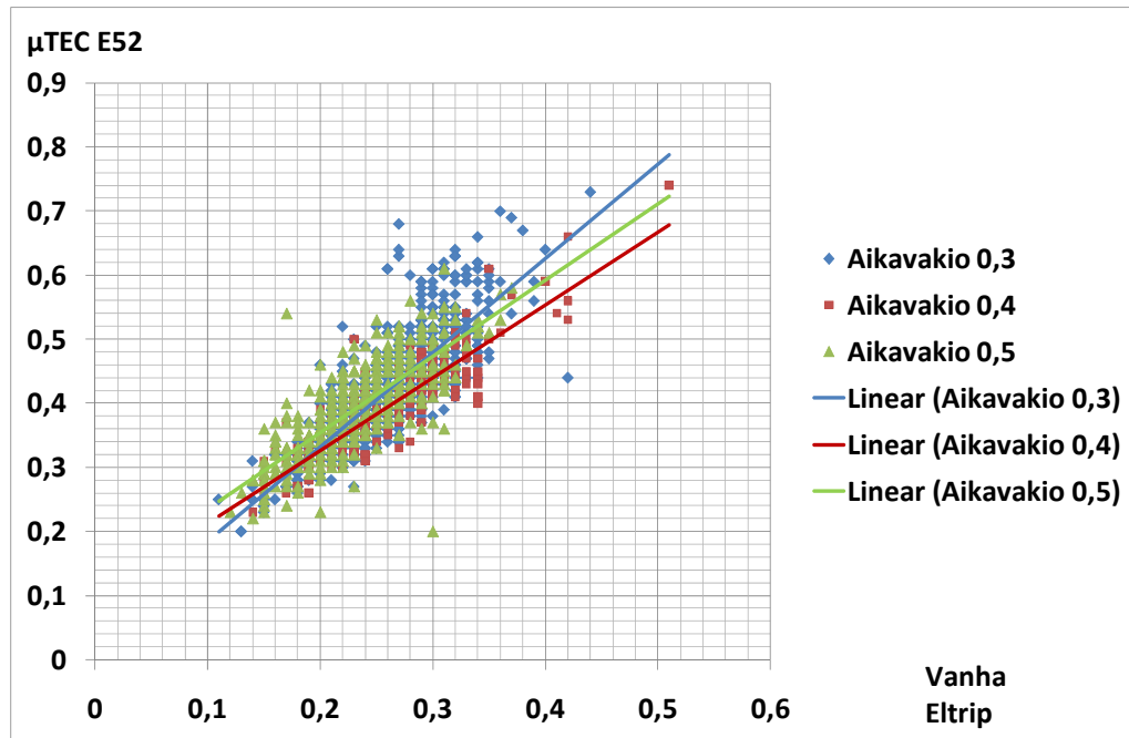
Kuva 31. E52-matkapuhelimeen ladatun \mu TEC:in ja vanhan Eltripin vertailua. "Aikavakio 0,3" tarkoittaa ajanjaksoa 2.2.–28.2., jolloin \mu TEC:ien aikavakio oli 0,3. "Aikavakio 0,4" tarkoittaa ajanjaksoa 7.3.–13.3., jolloin aikavakio oli 0,4. "Aikavakio 0,5" tarkoittaa ajanjaksoa 24.3.–29.3., jolloin aikavakio oli 0,5.
