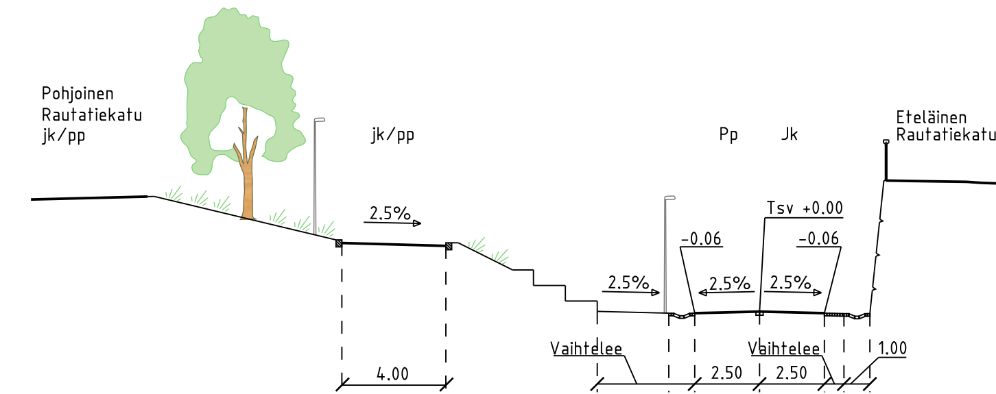
POIKKILEIKKAUS D-D
