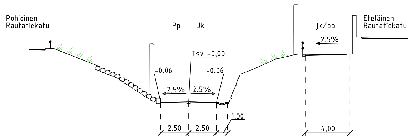
POIKKILEIKKAUS F-F
