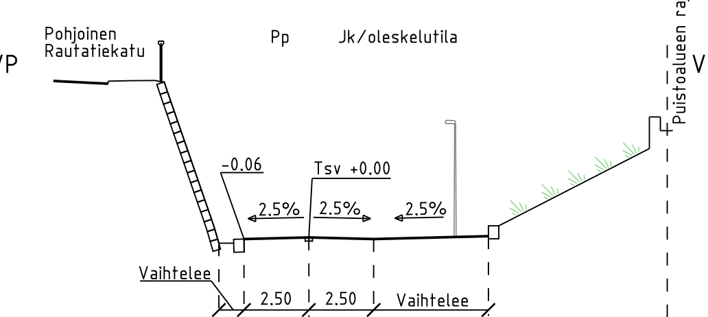
POIKKILEIKKAUS K-K
