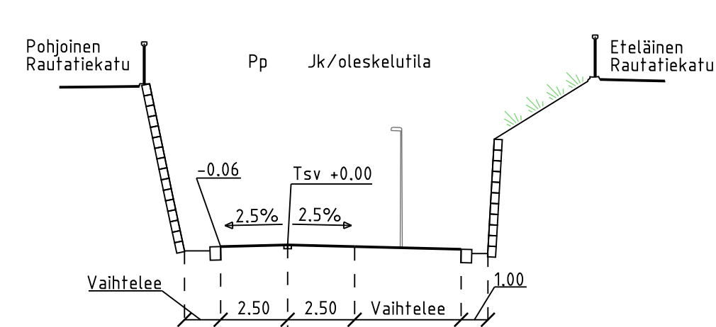
POIKKILEIKKAUS H-H
