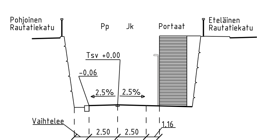
POIKKILEIKKAUS G-G
