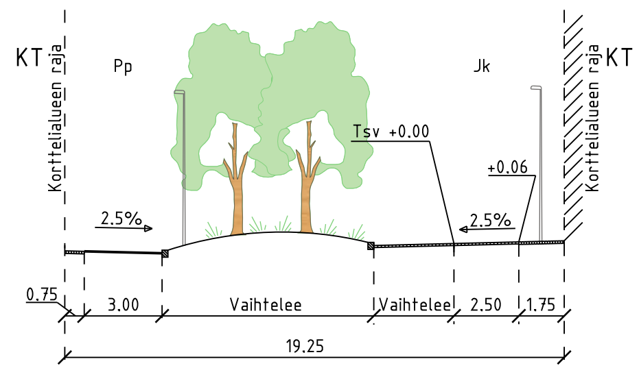
POIKKILEIKKAUS A-A
