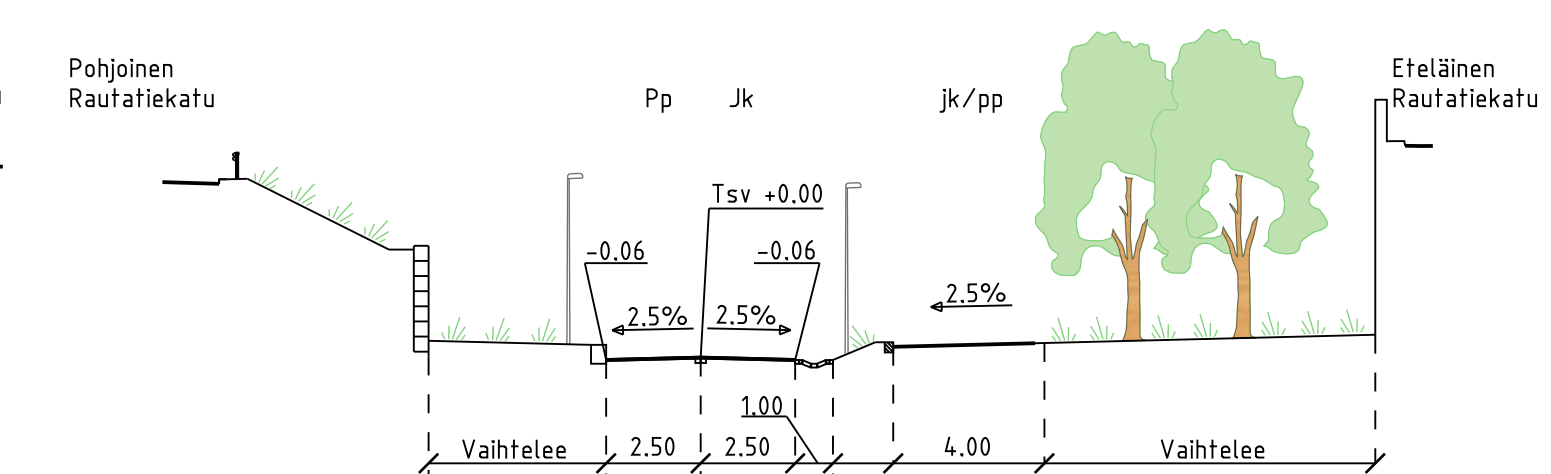
POIKKILEIKKAUS E-E
