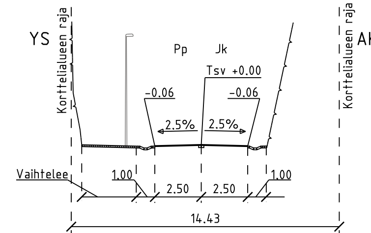
POIKKILEIKKAUS C-C
