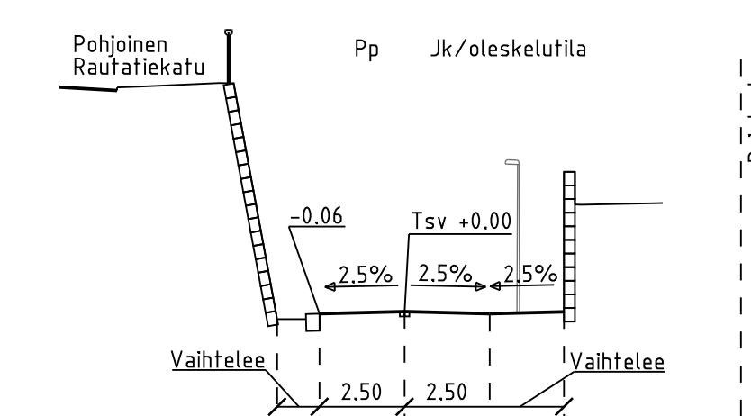
POIKKILEIKKAUS J-J
