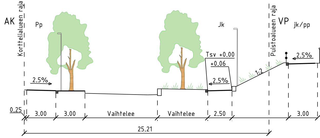
POIKKILEIKKAUS B-B
