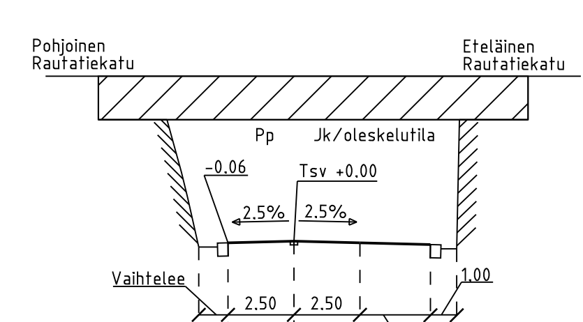
POIKKILEIKKAUS I-I
